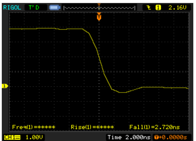
Рис.7 Задний фронт на нагрузке 150 Ом.
