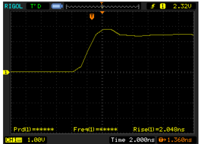
Рис 5 Передний фронт на нагрузке 50 Ом.
