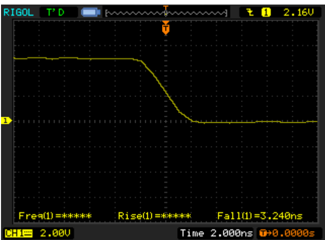
Рис.6 Задний фронт импульса без нагрузки.
