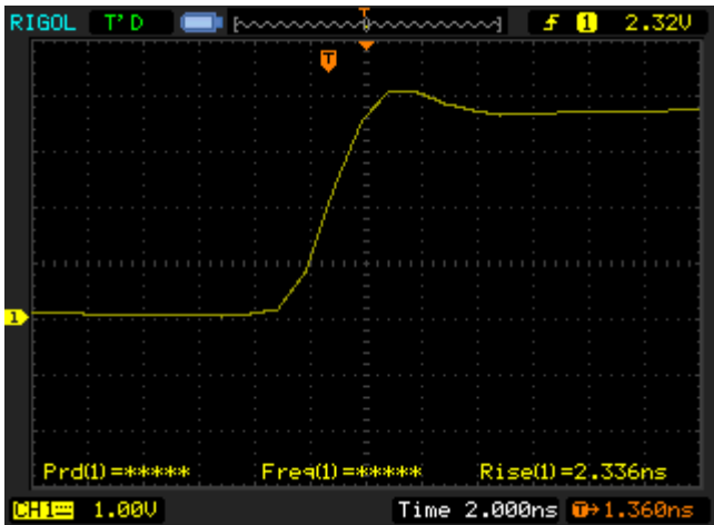
Рис.4 Передний фронт на нагрузке 150 Ом.
