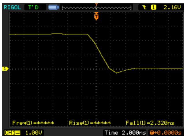
Рис.8. Задний фронт на нагрузке 50 Ом.
