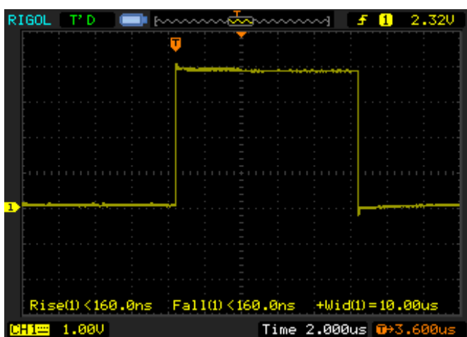
Рис.2 Длительность импульса.
