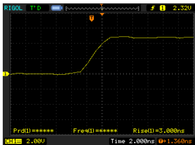
Рис.3 Передний фронт без нагрузки.
